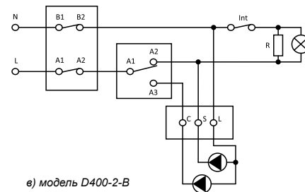
в) модель D400-2-B
