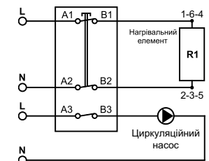
а) модель MIXTE DS PORT./DK – 230 В
